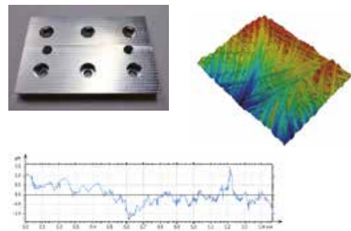
Metallityöstetty pinta (alumiini)
